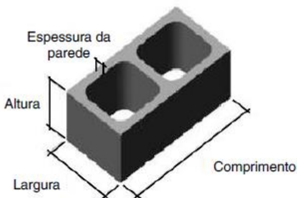
Figura 1 – Bloco vazado de concreto simples
