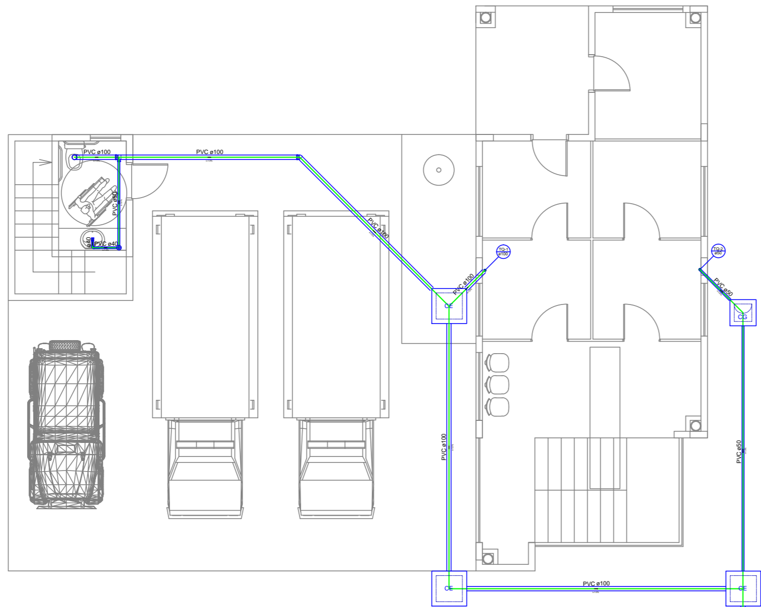
PLANTA BAIXA TERREO A= 61,69m 2 Escala: 1:75
