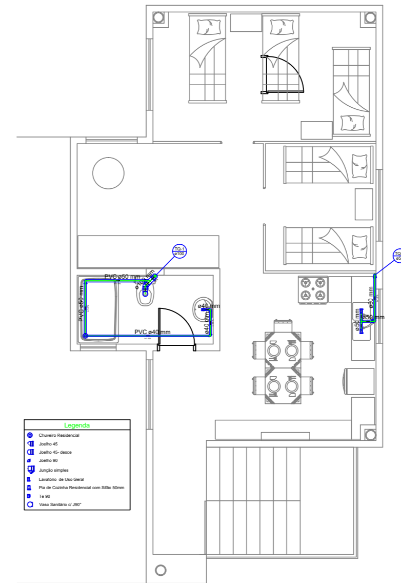
PLANTA BAIXA SUPERIOR A= 73,17m 2 Escala: 1:75
