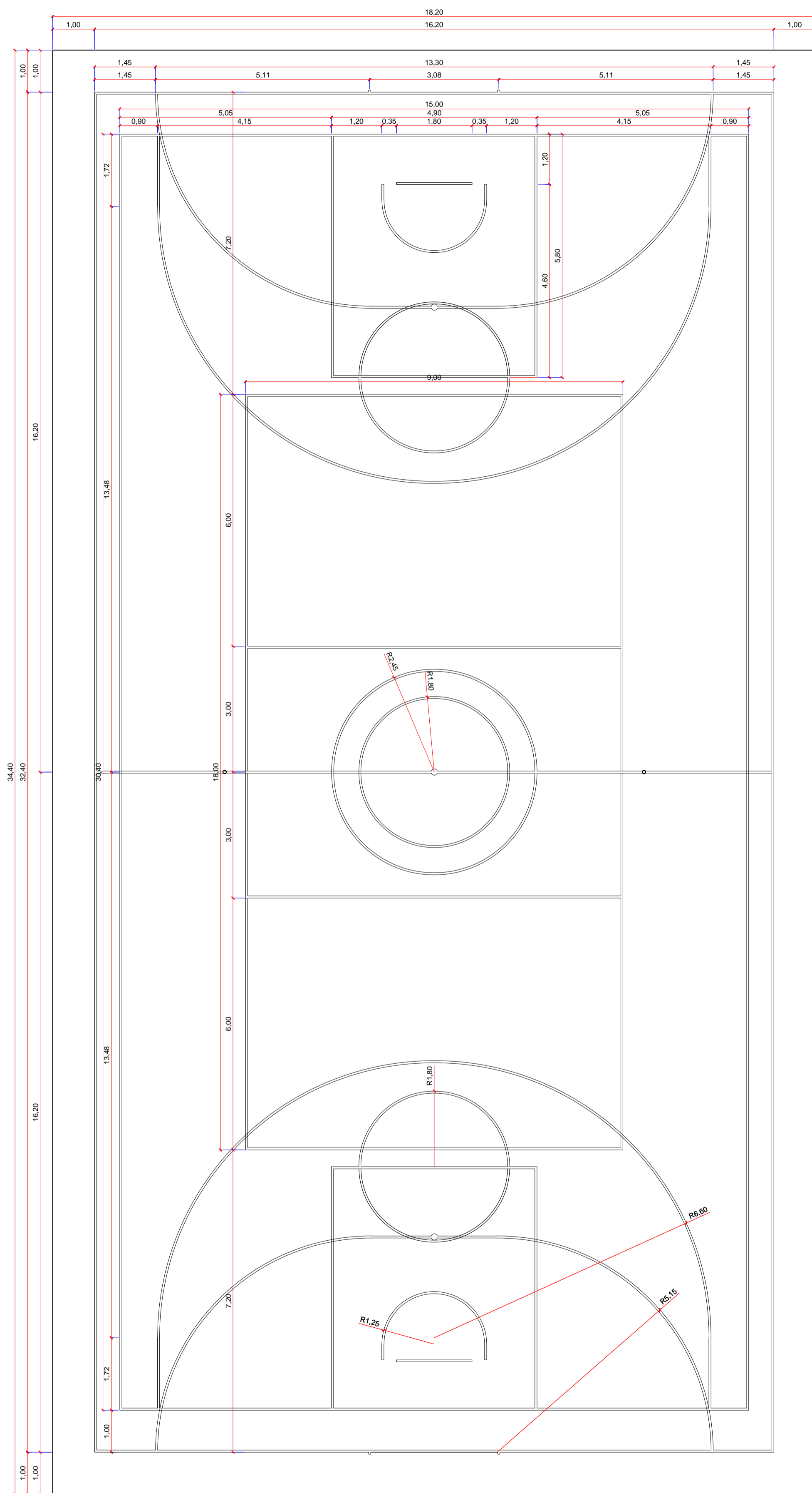
Marcação de faixas esc - 1/75 unidade metros
