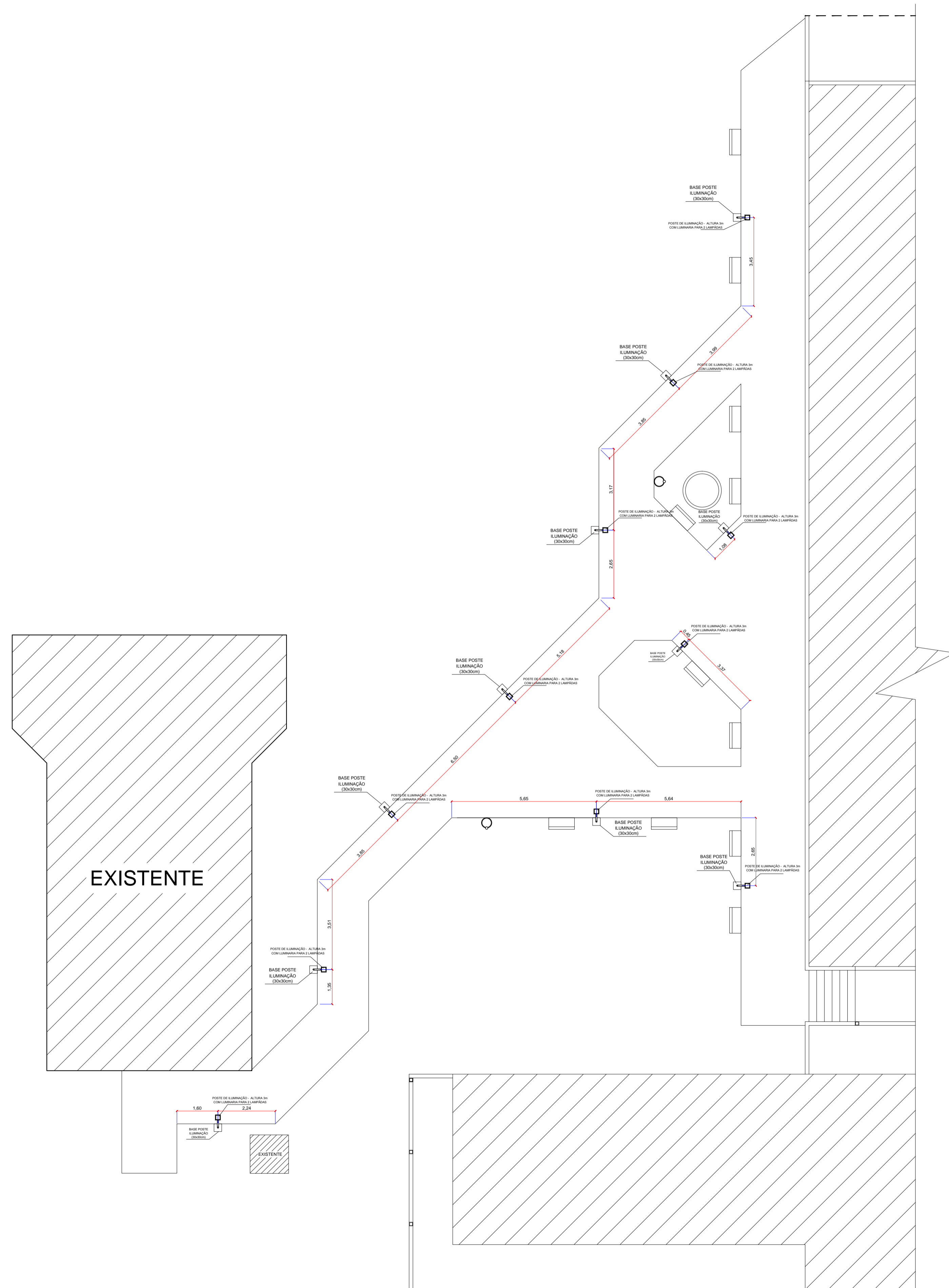
Planta baixa - Locação de poste de iluminação esc - 1/100 unidade metros
