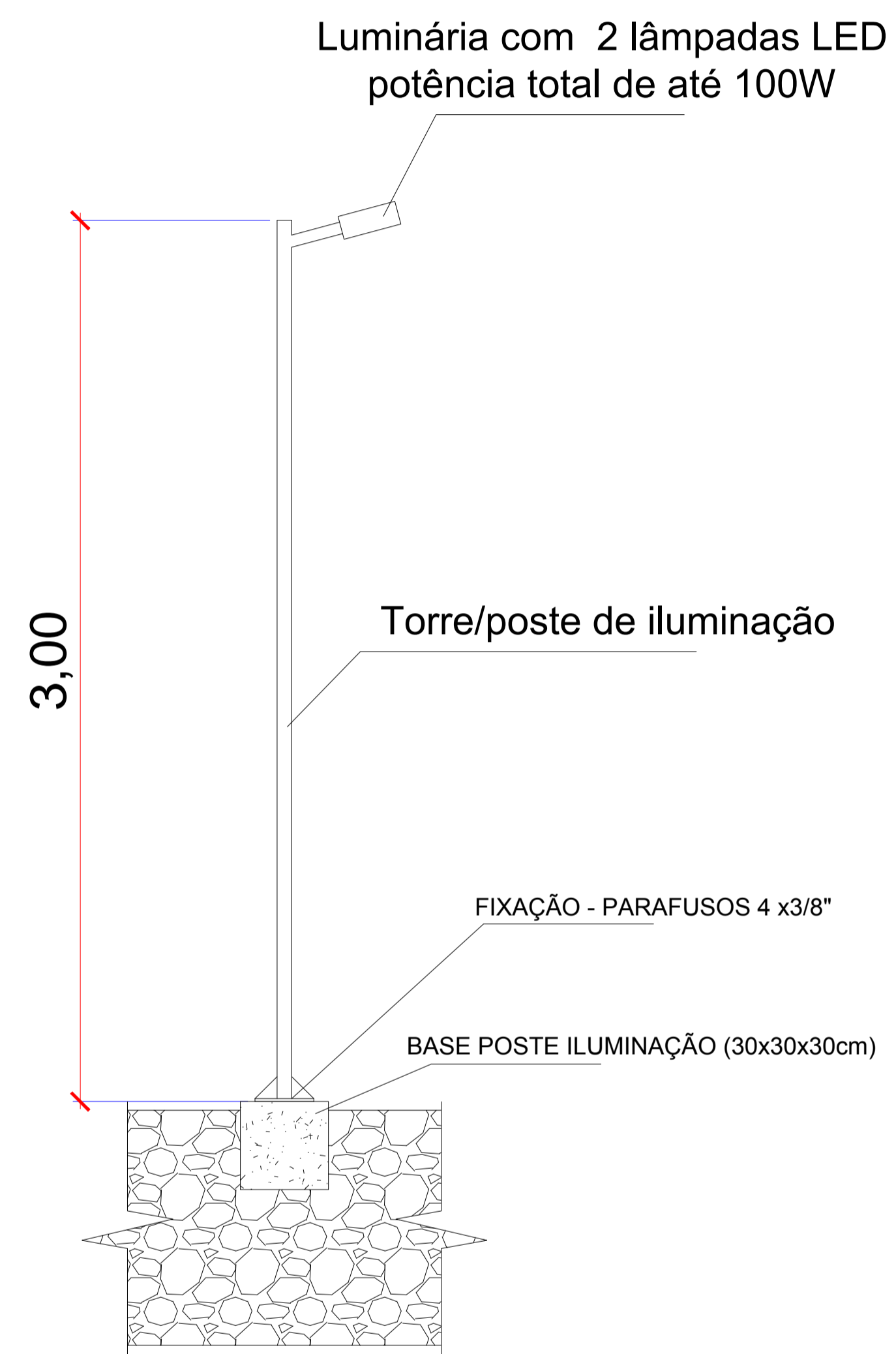
DETALHE POSTE DE ILUMINAÇÃO SEM ESCALA
