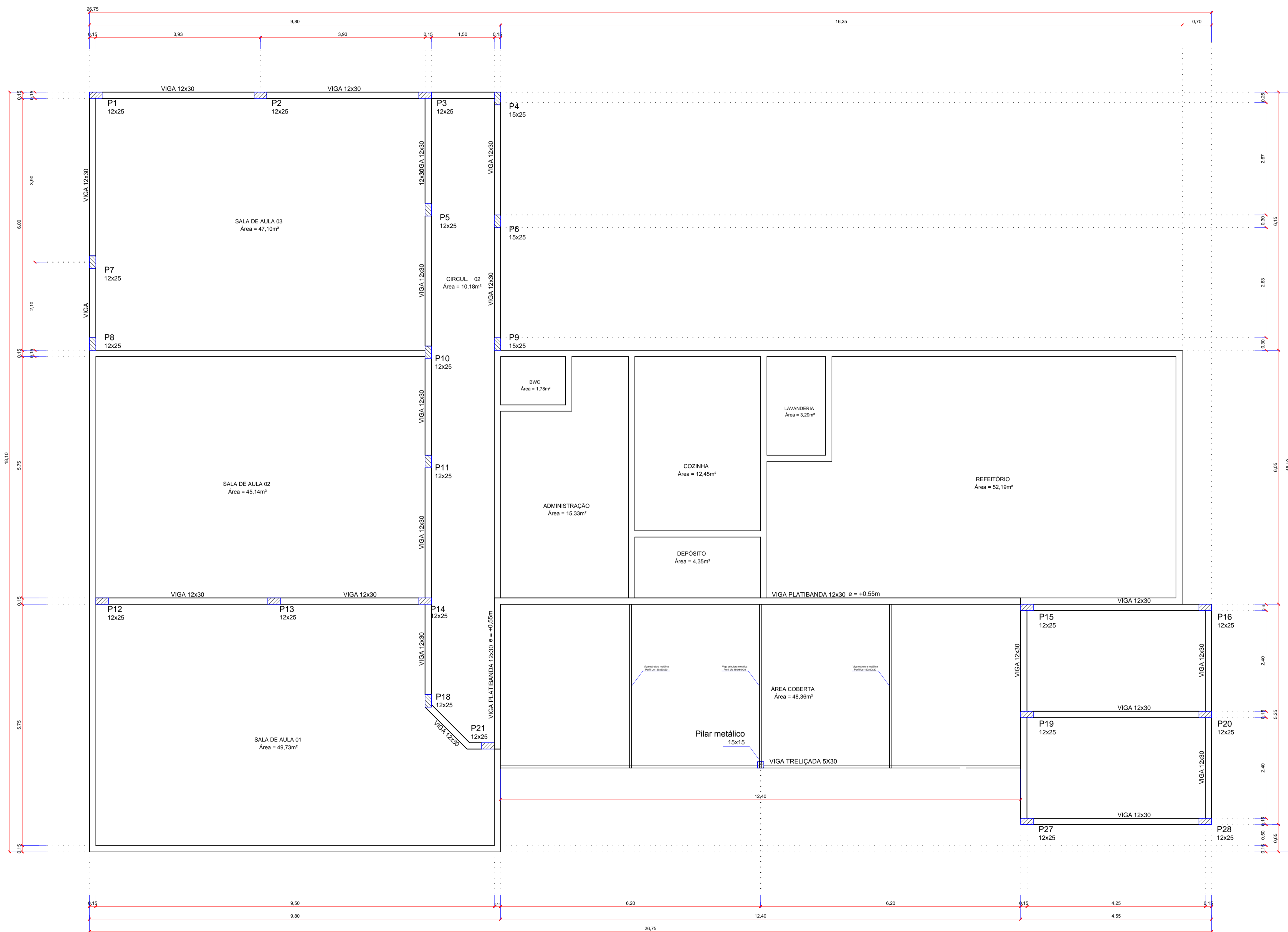
FORMA COBERTURA (Nível +3,00 e +3,05) escala 1:50
