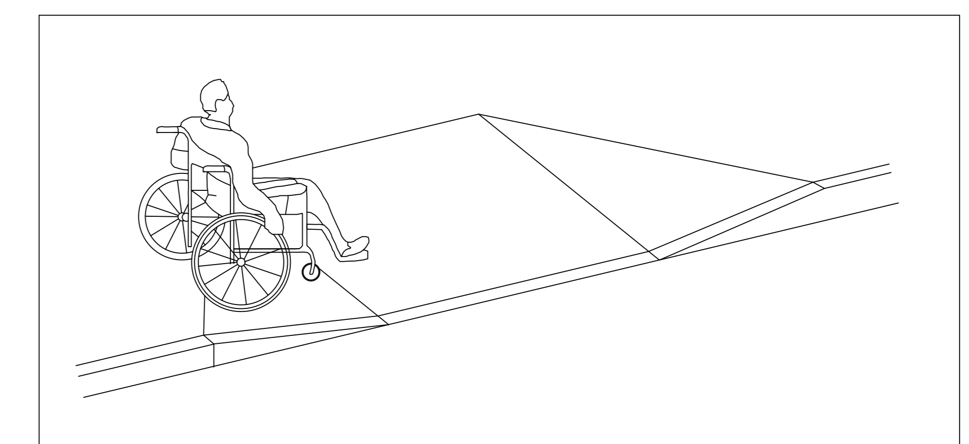
RAMPA ACESSIBILIDADE ESCALA: S/E
